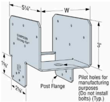
EPCZ End Post Cap
